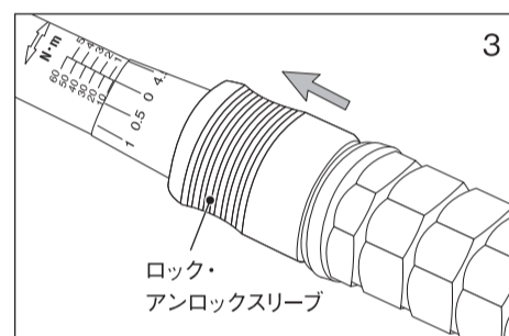
主目盛り30N・m+a 副目盛り2N・m 主目盛り30N・m+副目盛り2N・m=設定値32N・m
