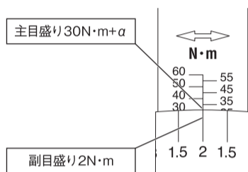
主目盛り30N・m+a 副目盛り2N・m 主目盛り30N・m+副目盛り2N・m=設定値32N・m
