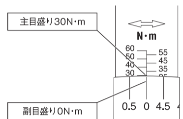
主目盛り30N・m 副目盛り0N・m 主目盛り30N・m+副目盛り0N・m=設定値30N・m
