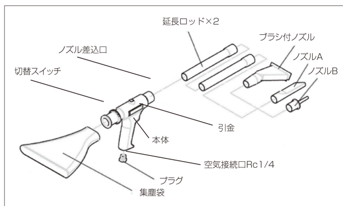
図1 各部名称
