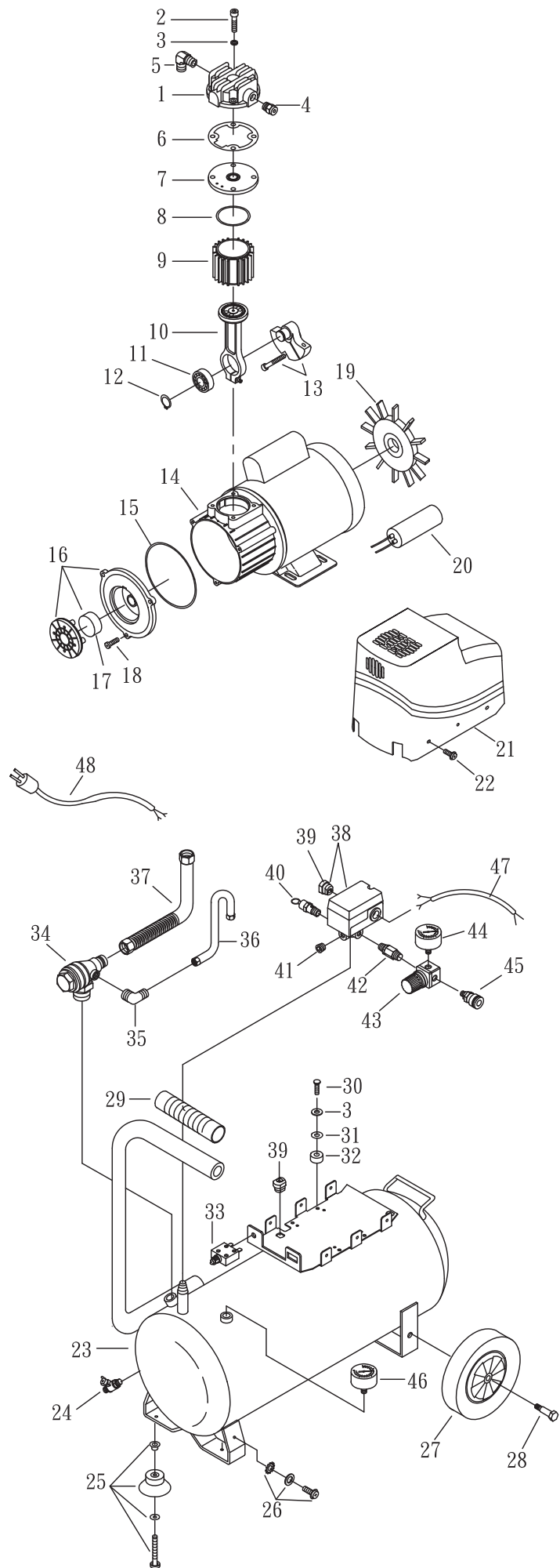
SR-102 分解図
