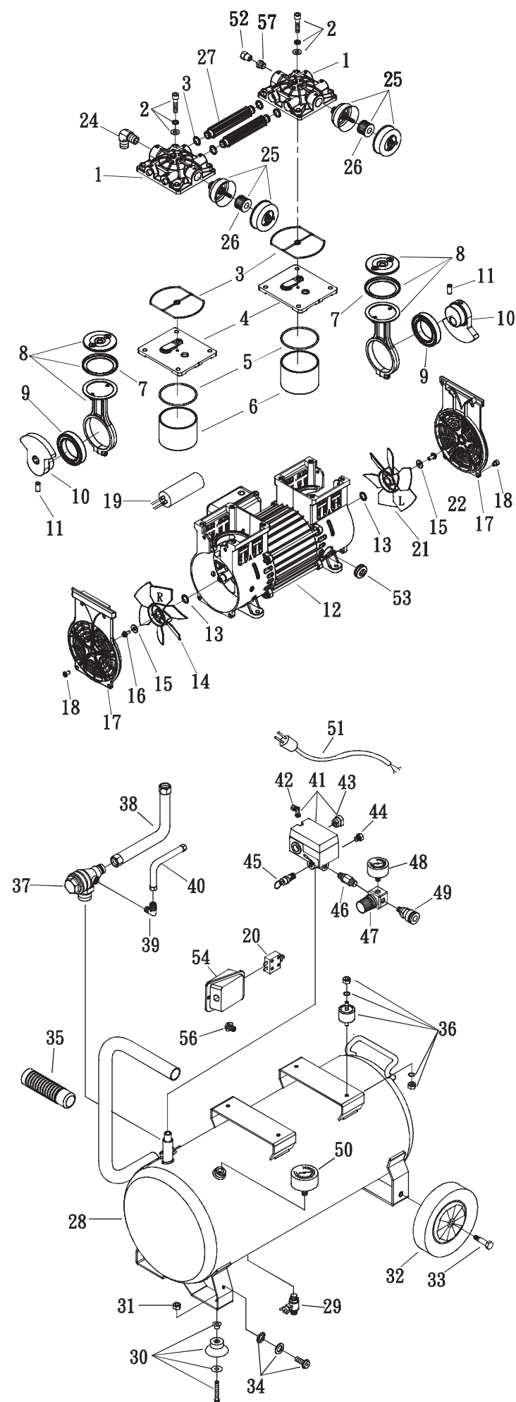
SW-231 分解図
